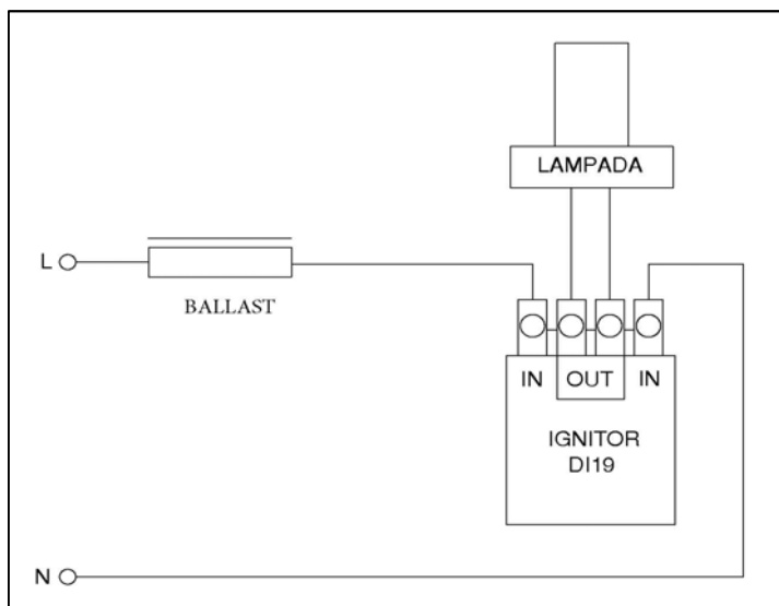
Diagramma di collegamento/Wiring diagram
